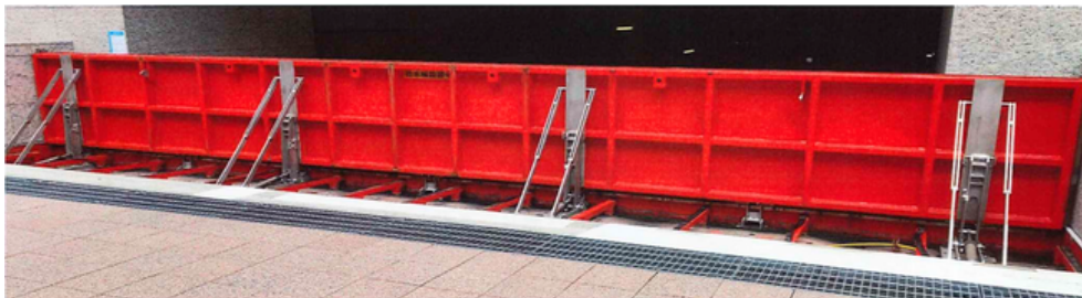
脱着式
